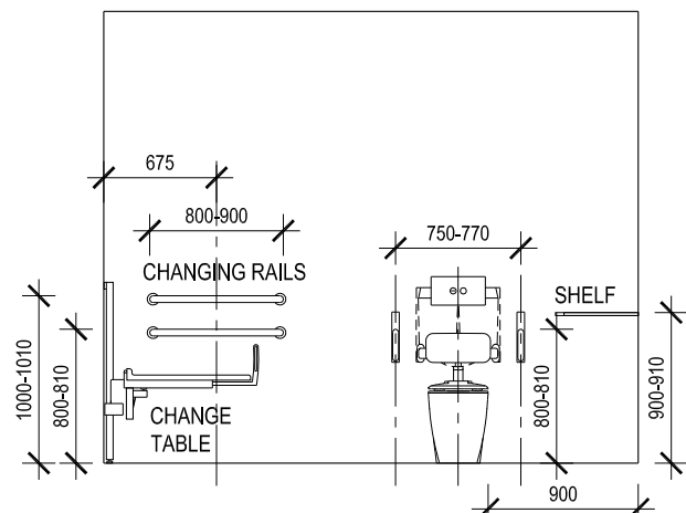
ELEVATION A
