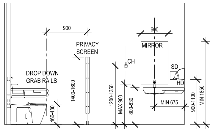
ELEVATION B
