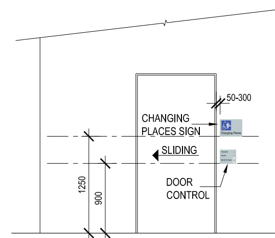
EXTERNAL DOOR
